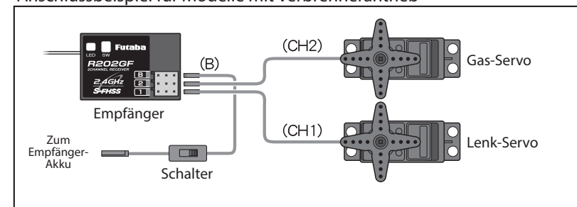
Anschlussbeispiel für Modelle mit Verbrennerantrieb
